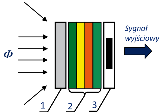
Rys. 3. Elementy składowe typowej głowicy fotometrycznej luksomierza: 1 – element korekcji przestrzennej, 2 – zestaw filtrów absorpcyjnych korekcji widmowej, 3 – detektor
